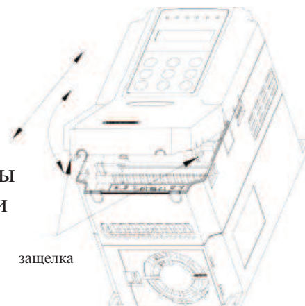
Рис.3-4 Демонтаж и сборка металлической крышки
