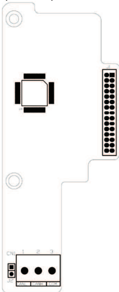
Рис. D-2 Габаритный чертеж CANopen
