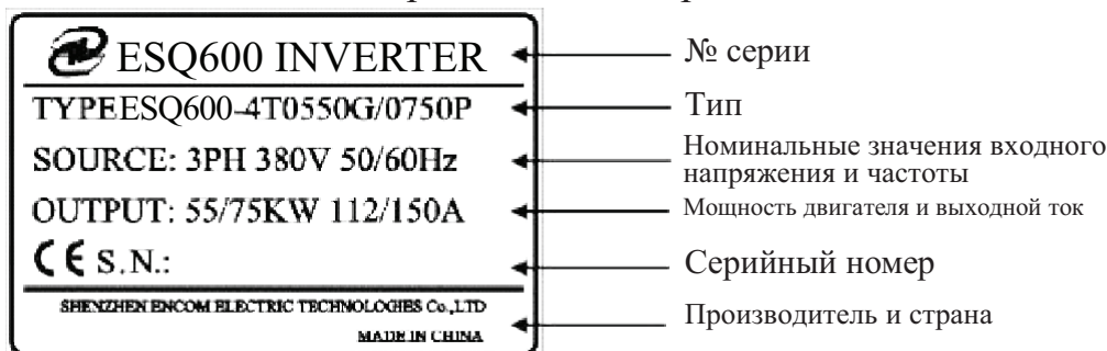
Рис.2-2 Заводская табличка
