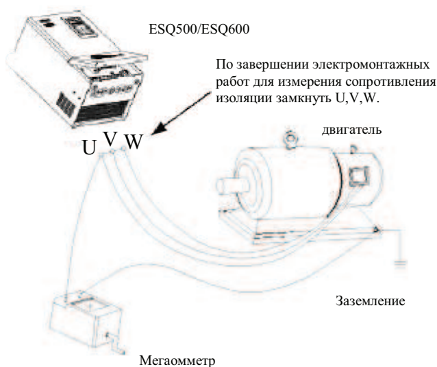
Рис.1-1 Контроль изоляции двигателя
