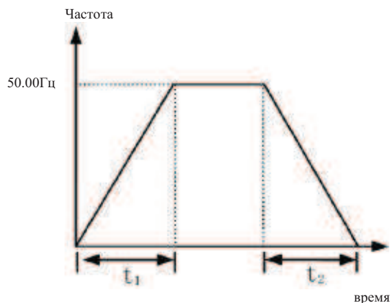
Рис. 7-1 Линейное ускорение и замедление
