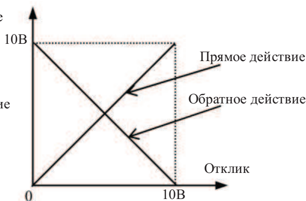
Рис.7-41 Характеристики отклика
