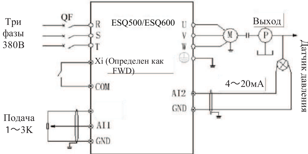
Рис.7-36 Схема системы управления со встроенным ПИД -регулятором
