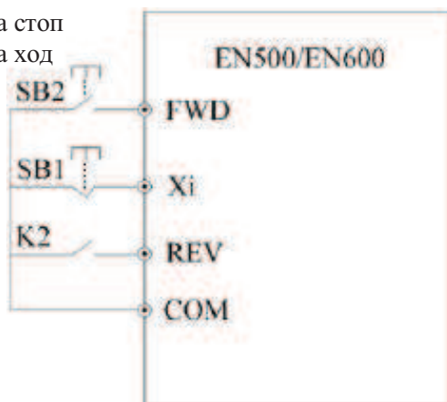
Рис. 7-20 Трехпроводный режим управления 2
