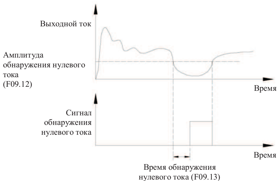
Рис.7-26 Диаграмма обнаружения нулевого тока
