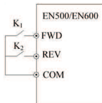
Рис. 7-17 Двухпроводный режим управления 2
