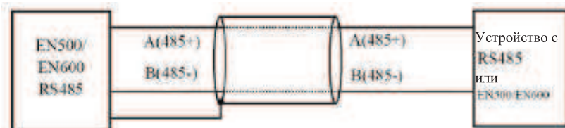
Рис .3 -18 Монтаж разъема передачи данных
