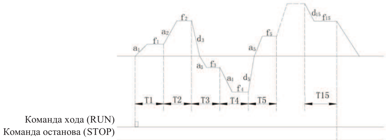
Рис.7-31 Остановка работы после одного цикла работы ПЛК
