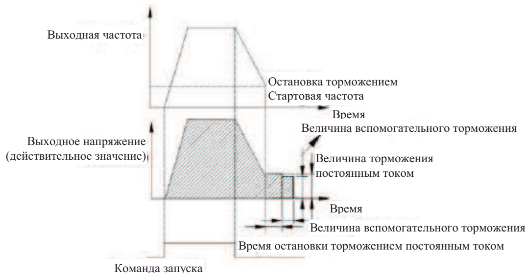
Рис. 7-5 Остановка с замедлением + Торможение постоянным током
