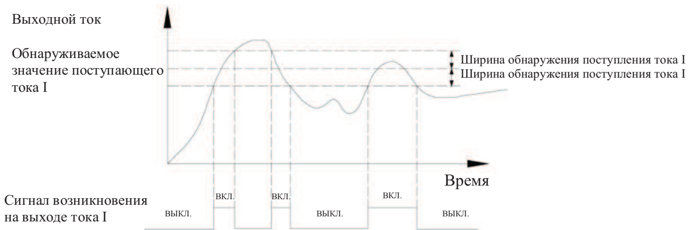
Рис.7-28 Схема обнаружения поступающего тока
