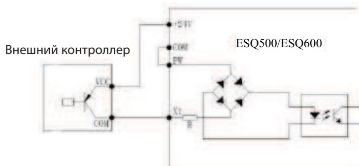
Рис. 3-15 Режим подключения со стоком на 24В 2. Для использования внешнего источника питания 5~30В постоянного тока и режима подключения внешнего контроллера типа NPN-исток (уберите короткозамыкающую пластину между клеммами PW и +24V).
