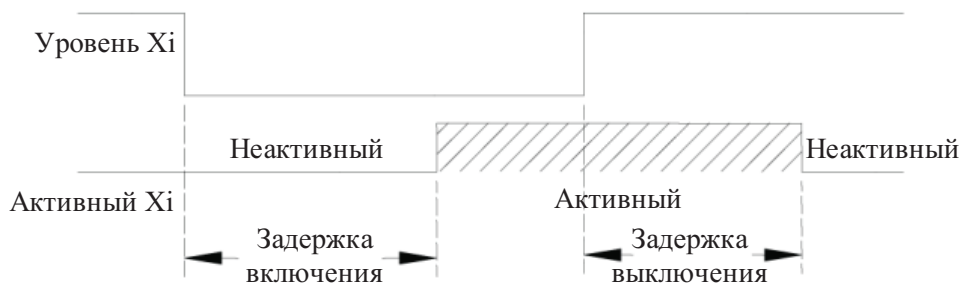
Рис. 7-13 Задержка открытия и закрытия
