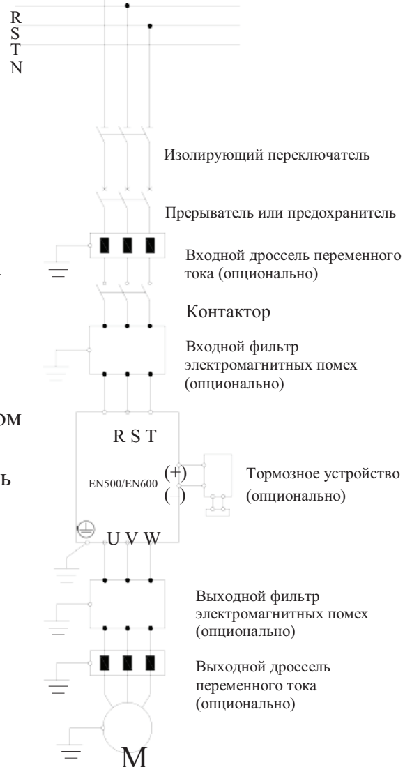
Рис.3-8 Соединение преобразователя и сопрягаемых деталей
