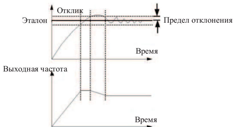
Рис.7-39 Предел отклонения
