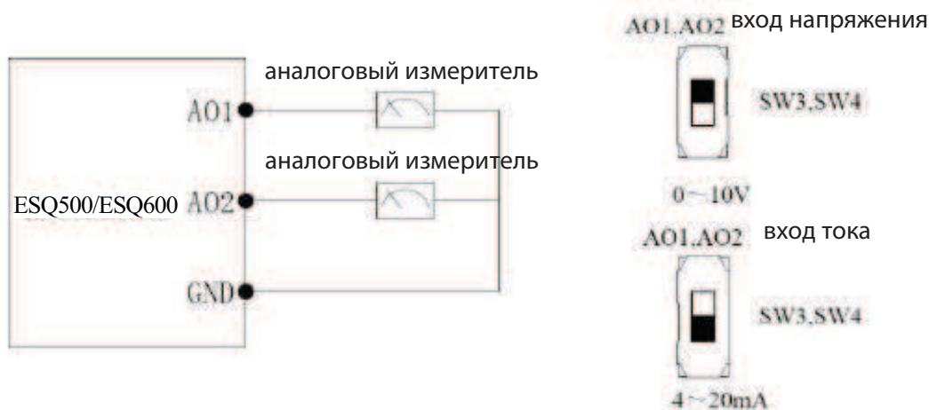
Рис.3-13 Схема монтажа клемм AO1, AO2
