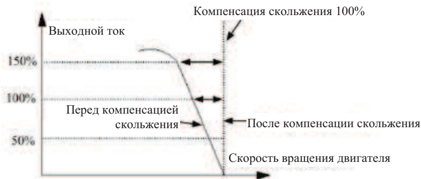
Рис. 7-10 Компенсация частоты скольжения
