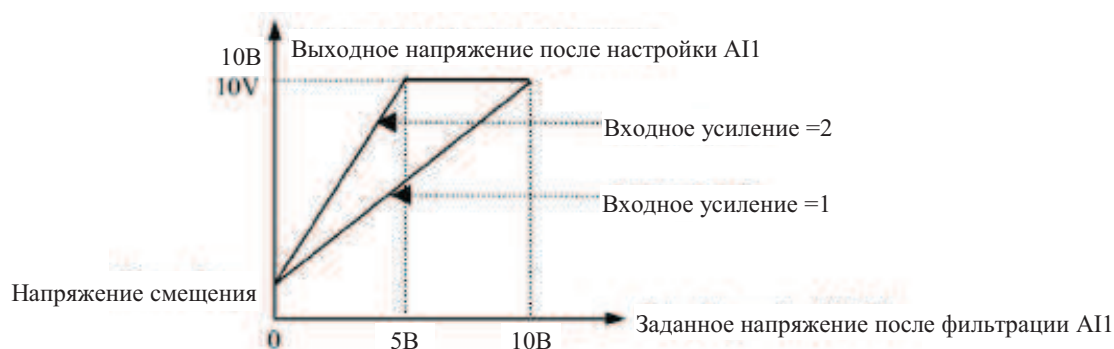
Рис. 7-12 Настройка AI1
