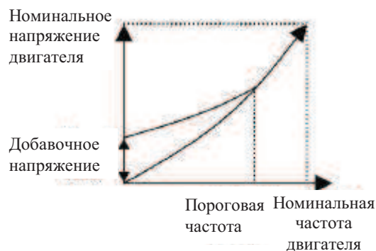
а Кривая понижения момента при форсировании момента
