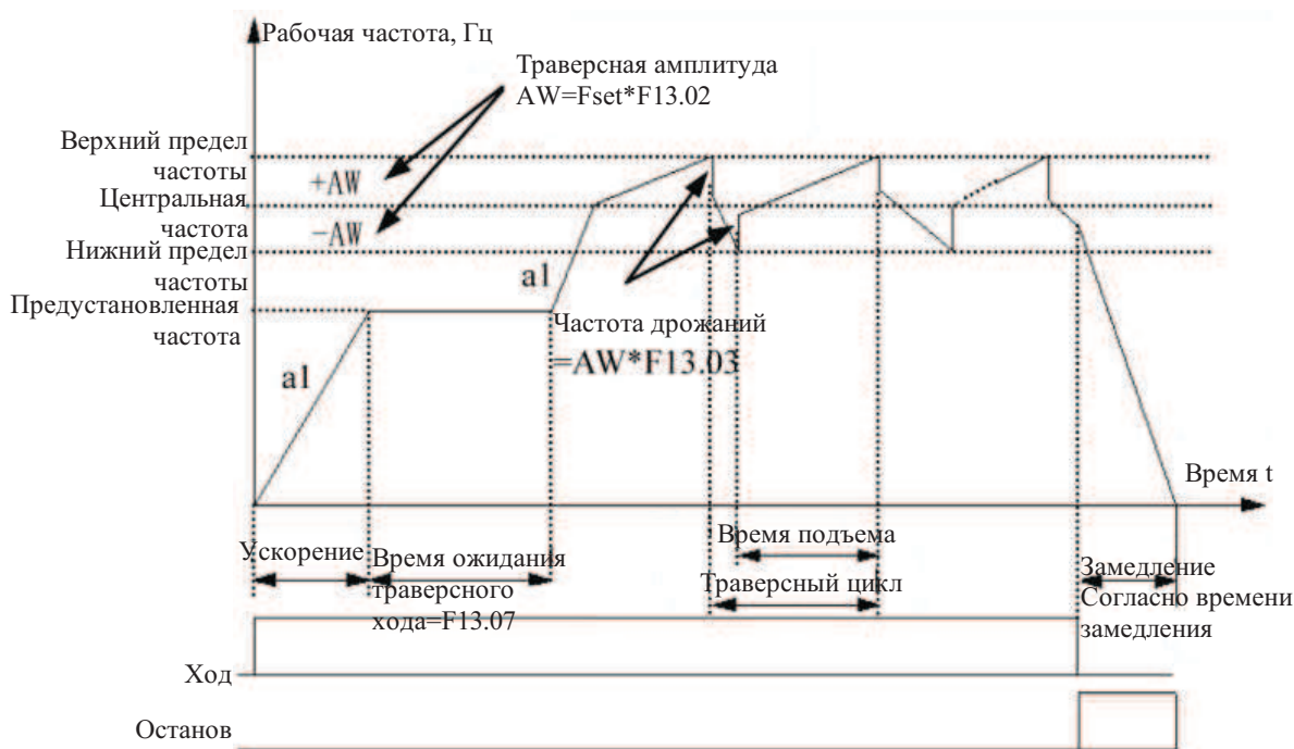
Рис.7-43 Траверсный ход
