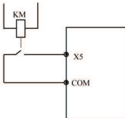
Рис. 7-15 Нормально открытый канал ошибки периферических устройств
