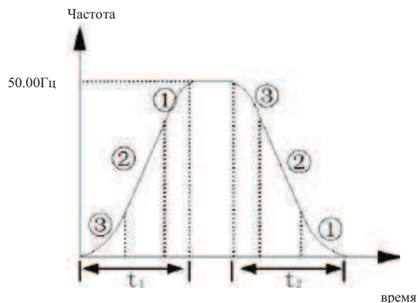
Рис. 7-2 Ускорение и замедление по S-кривой
