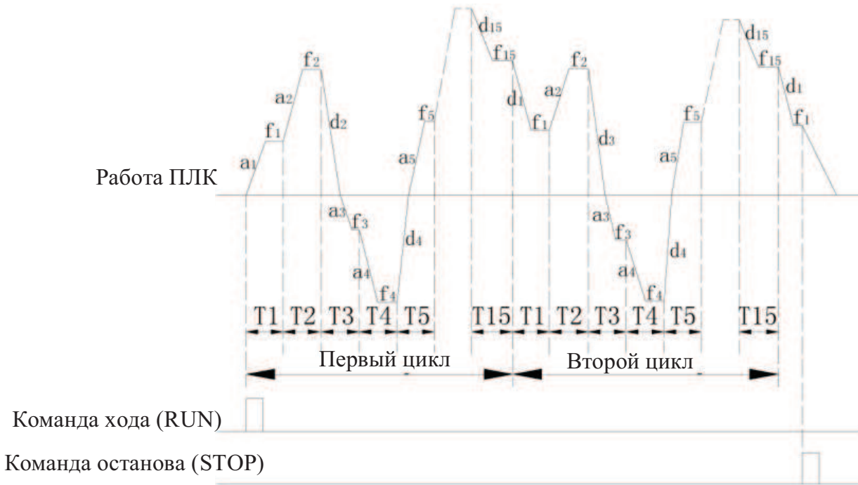
Рис 7-33 Непрерывный режим работы ПЛК
