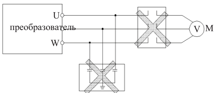
Рис.3-6 Запрещено использовать пускатель и поглощающий конденсатор
