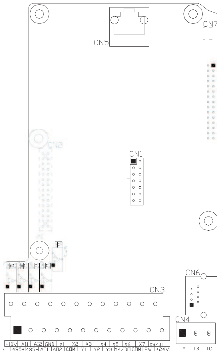
Рис.3-10 Эскизное представление платы центрального процессора
