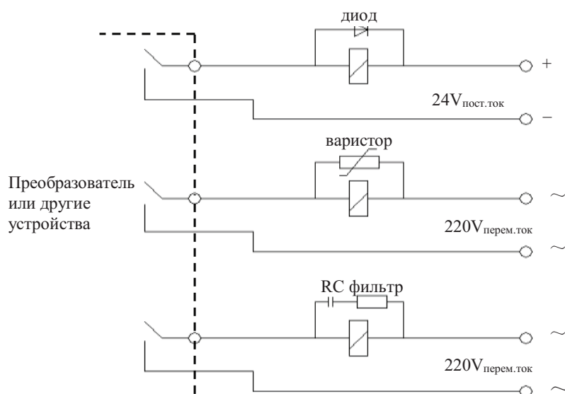
Рис.4-3 Требования к установке электромагнитного двухпозиционного электронного устройства
