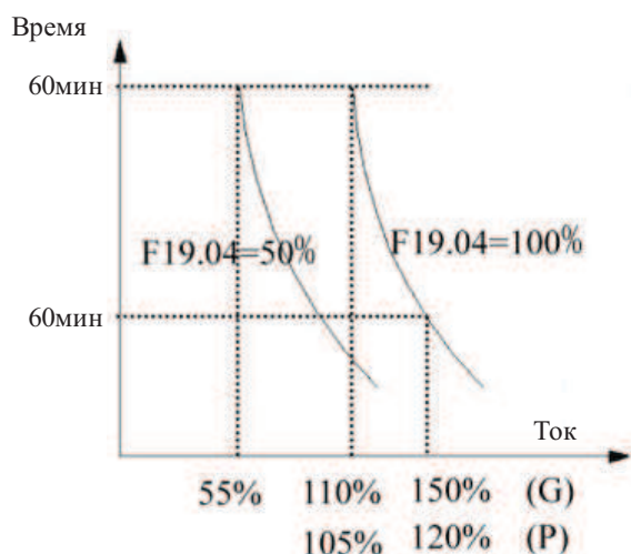
Рис.7-44 Защита электронным тепловым реле
