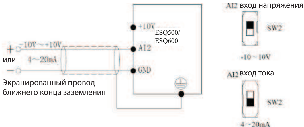
Рис. 3-12 Схема монтажа клеммы AI2
