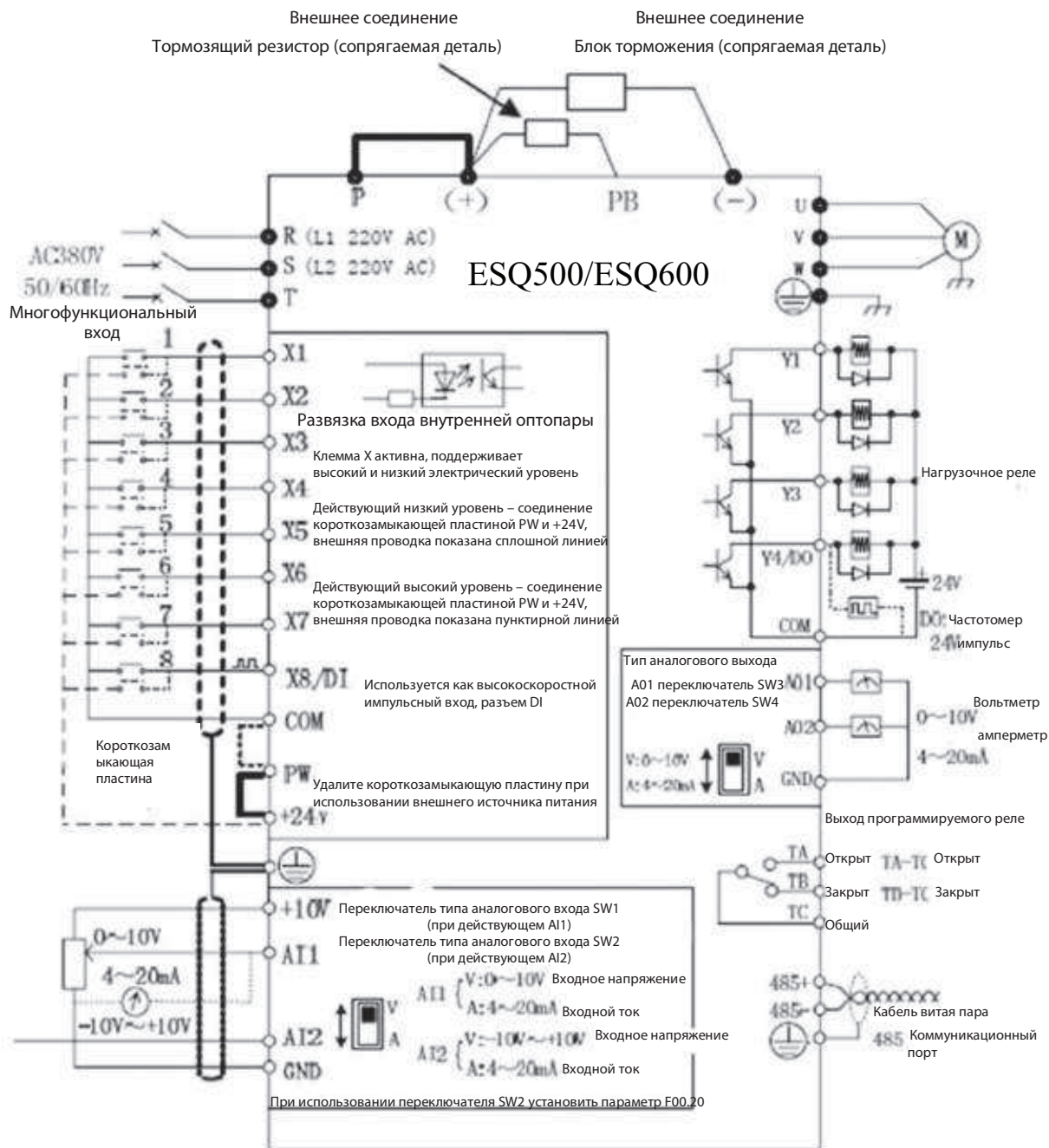
Рис. 3 -9 Базовая схема электрических соединений
