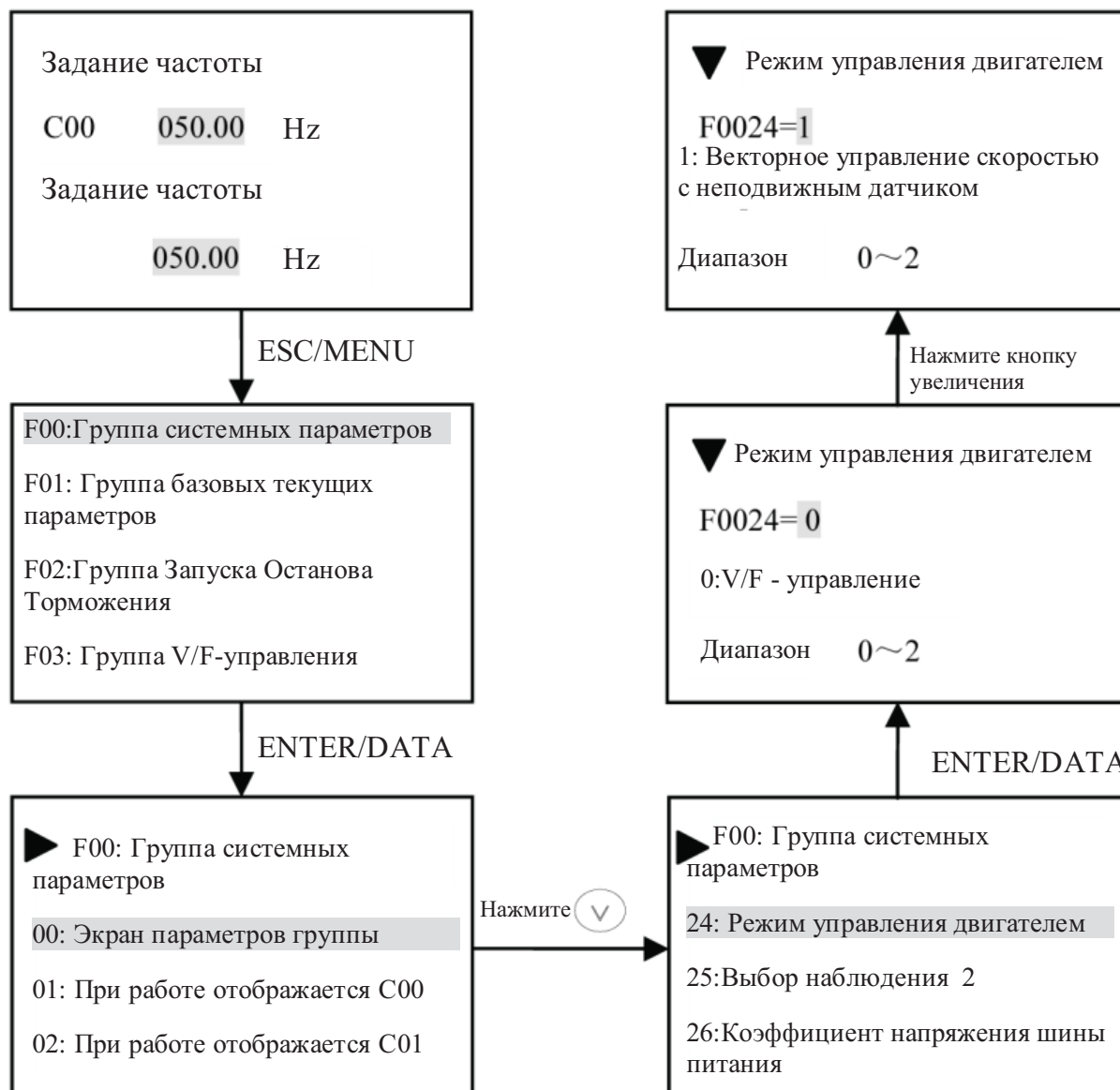
Рис.С-6 Пример редактирования параметров функций
