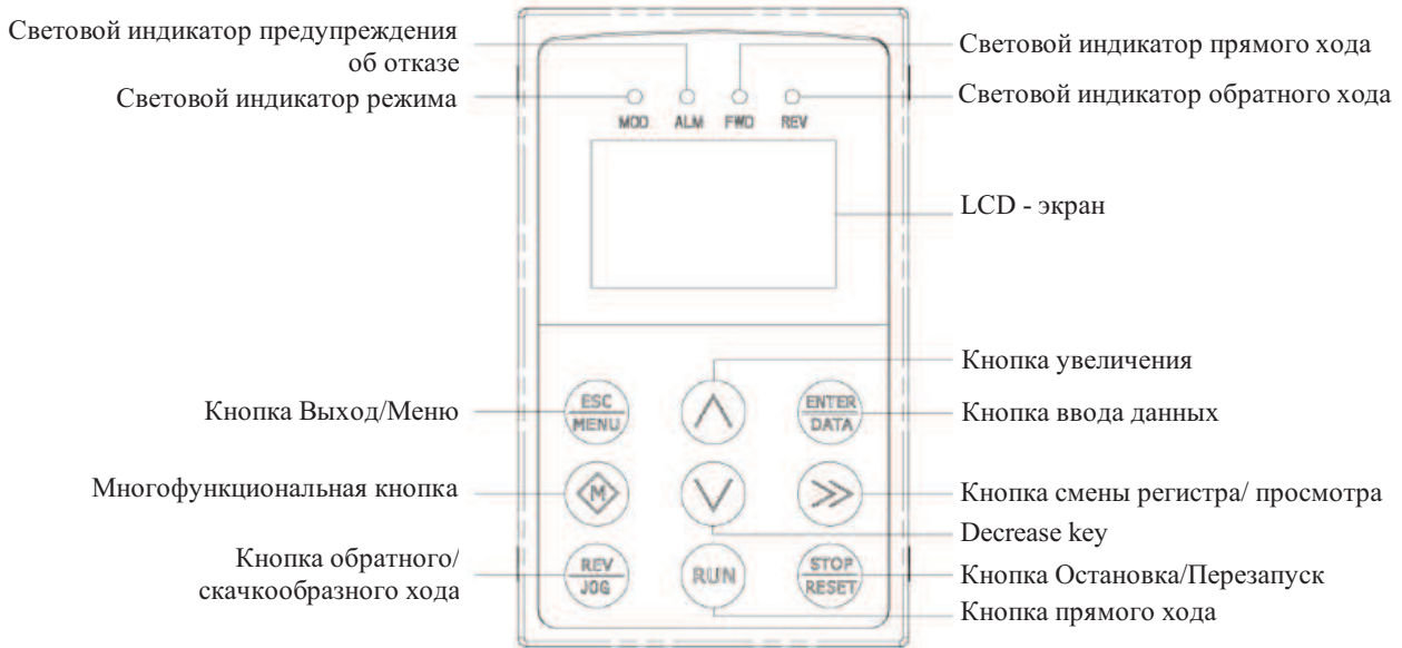
Рис.С-2 Схема пульта (EN-LCD1, EN-LCD2)
