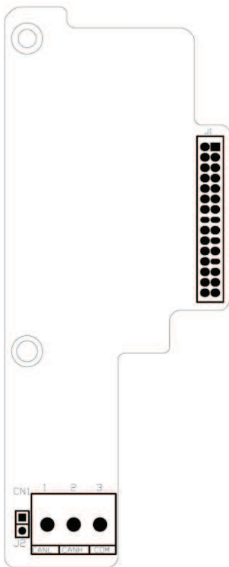
Рис. D-3 Размеры CANlink
