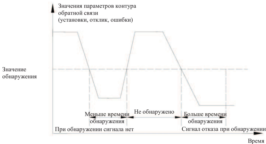
Рис. 7-48 Временная диаграмма обнаружения обратной связи
