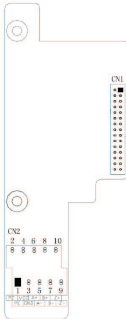
Рис.Е-1 Чертеж по габаритным размерам В-PG01, В-PG02
