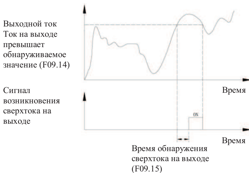
Рис.7-27 Схема обнаружения сверхтока на выходе
