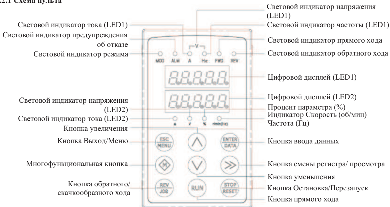
Рис.С-1 Схема пульта управления EN-LED2
