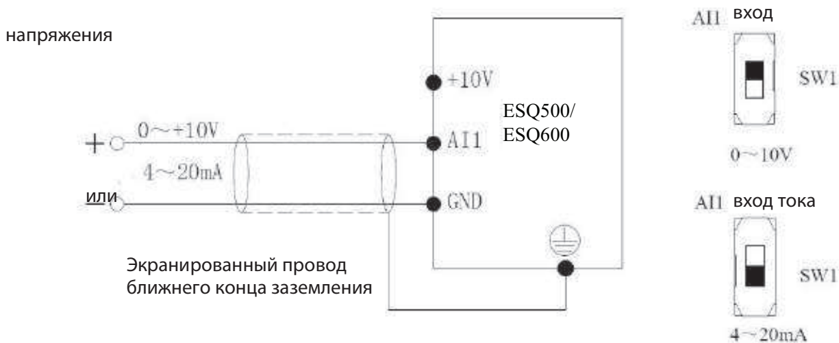
Рис.3-11 Схема монтажа клеммы AI1
