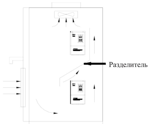
Рис.3-2 Установка нескольких преобразователей
