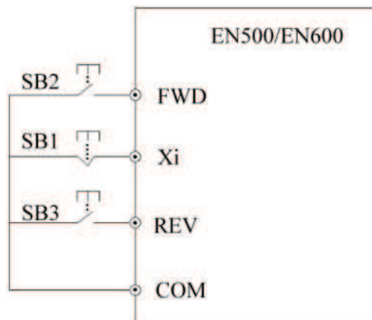
Рис. 7-19 Трехпроводный режим управления 1
