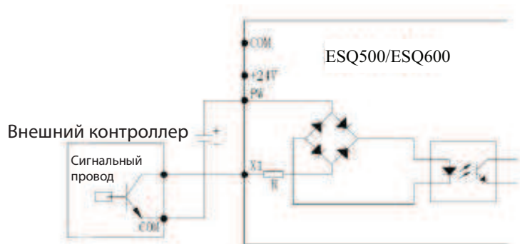
Рис.3-16 Режим подключения с внешним источником питания
