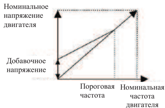
б Кривая постоянного момента при форсировании момента
