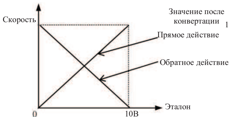
Рис.7-40 Характеристики системы с обратной связью
