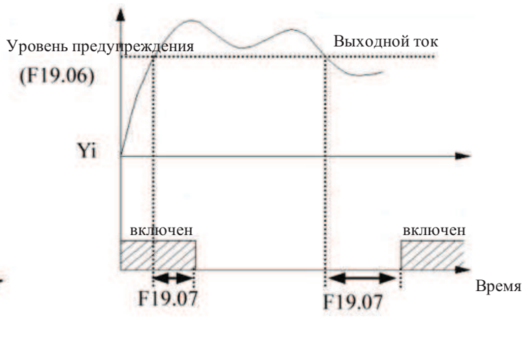
Рис.7-45 Сигнализация перегрузки
