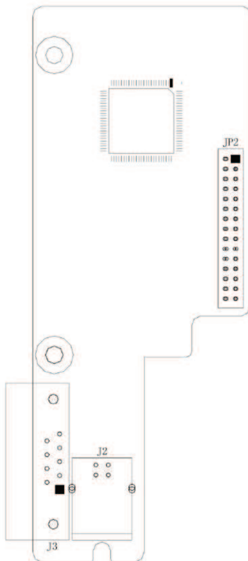
Рис. D-1 Габаритный чертеж PROFIBUS-DP
