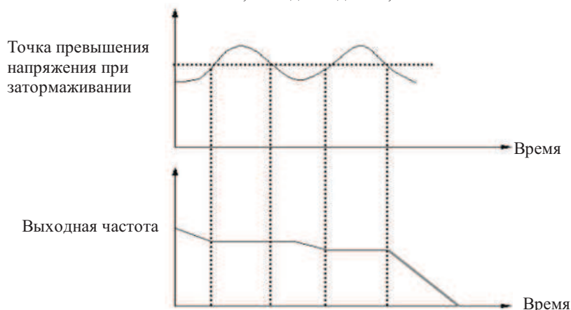
Рис. 7-46 Превышение напряжения при затормаживании
