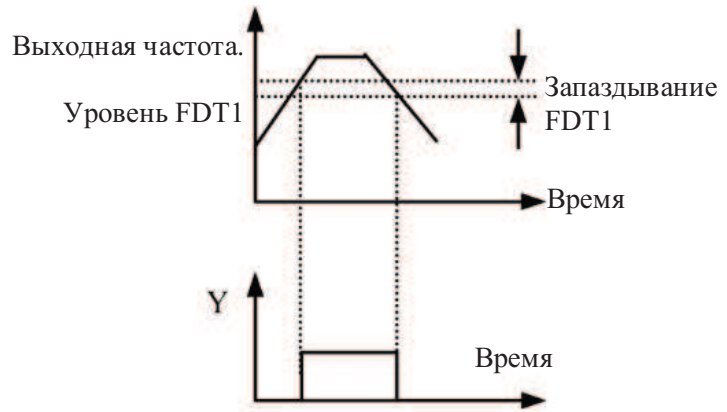
Рис.7-24 Диаграмма обнаружения частотного уровня
