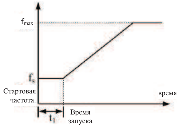
Рис. 7-3 Стартовая частота и время запуска
