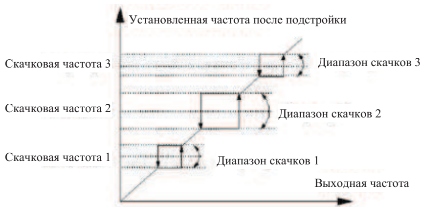
Рис. 7-9 Скачковые частоты и их диапазоны
