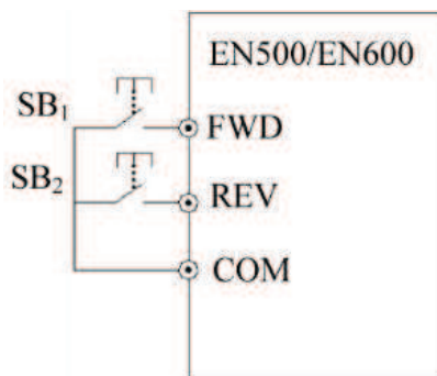
Рис. 7-18 Двухпроводный режим управления 3
