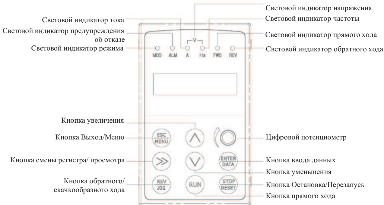
Рис.С-8 Схема пульта управления EN-LED3-D
