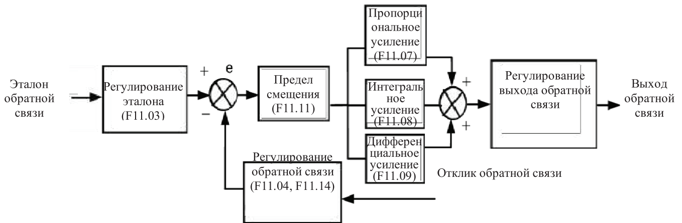
Рис.7-37 Схема принципа работы блока ПИД -регулирования
