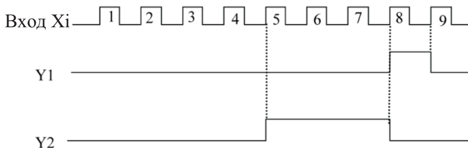
Рис. 7-21 Установка заданных и специальных значений внутреннего счетчика
