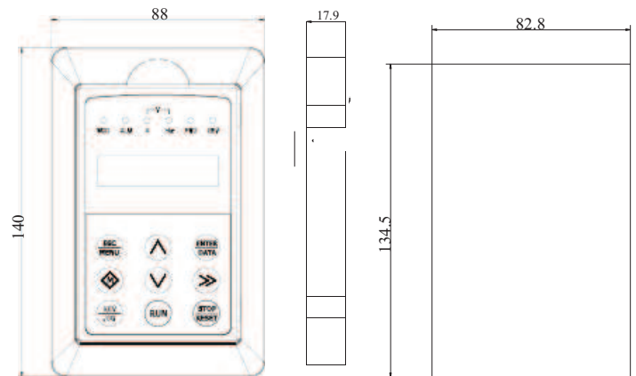
Рис.2-8 Габаритные размеры пульта управления
