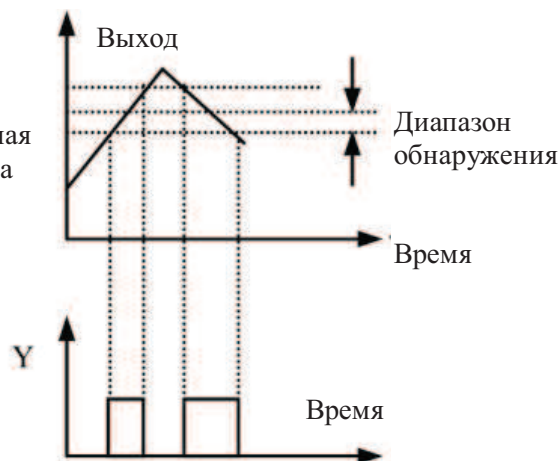
Рис.7-23 Диаграмма поступления частотного выходного сигнала
