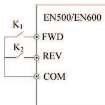
Рис. 7-16 Двухпроводный режим управления 1
