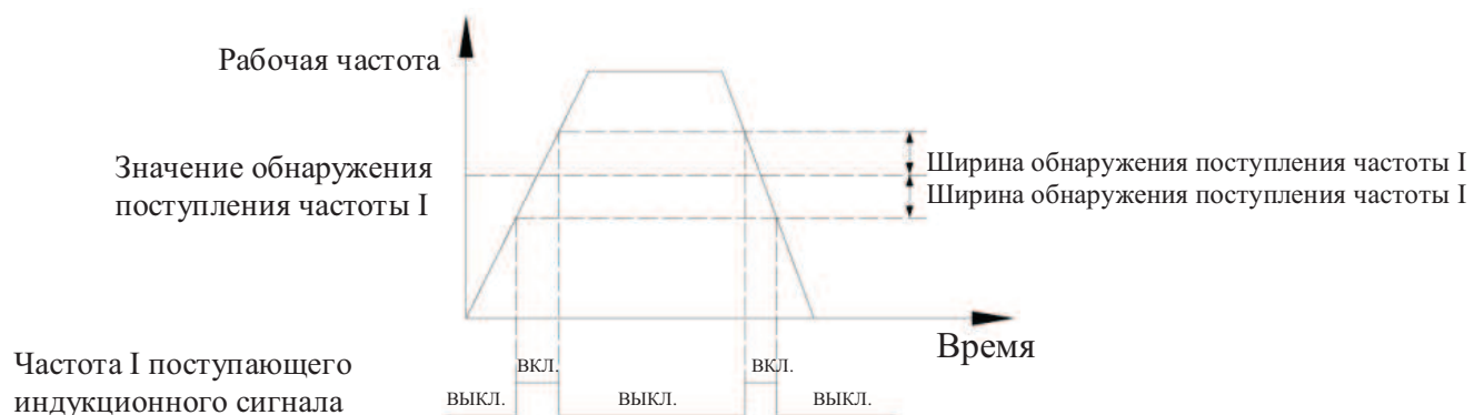
Рис.7-29 Диаграмма обнаружения поступления частотного сигнала
