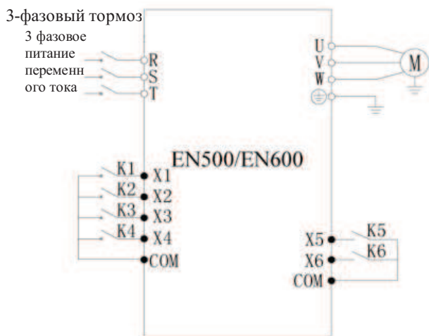
Рис. 7-14 Схема электрических соединений при режиме многоступенчатой скорости
