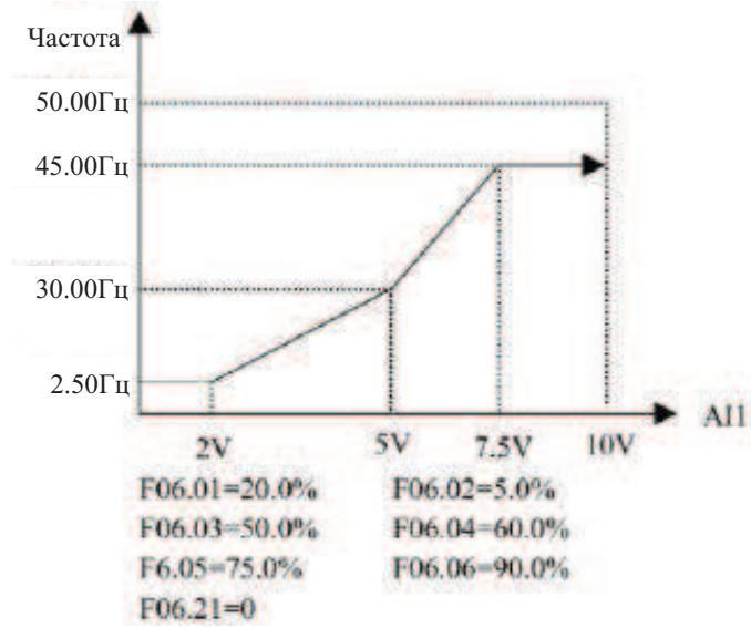
Рис. 7-11 АП выбирает установку частоты кривой 1
