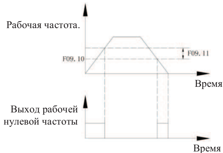
Рис.7-25 Обнаружение сигнала с нулевой частотой
