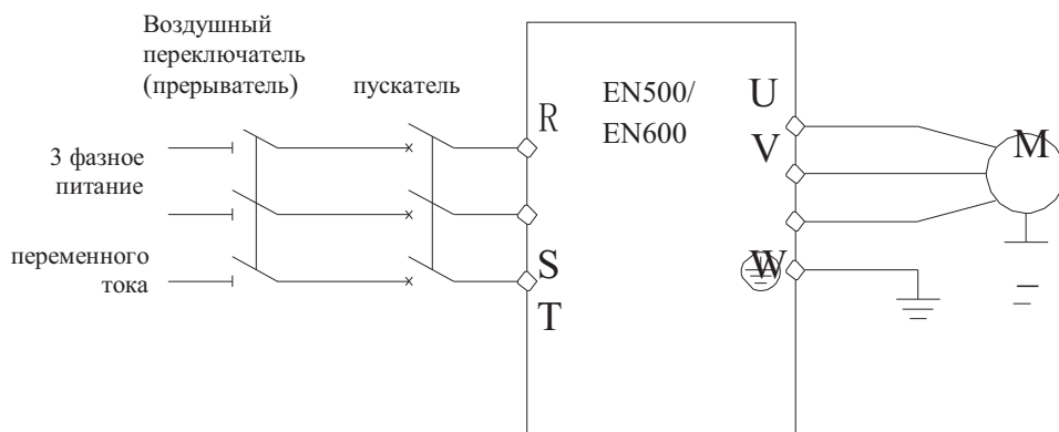
Рис.3-7 Простой монтаж основного контура
