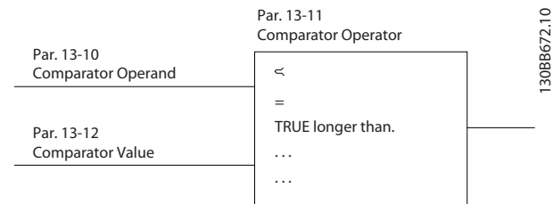
Рисунок 3.36 Компараторы
