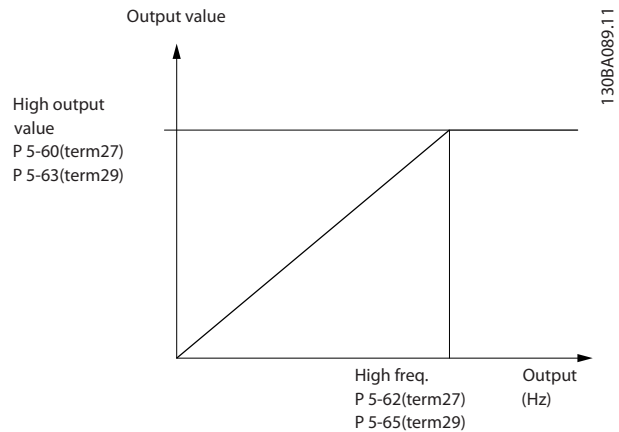
Рисунок 3.28 Импульсный выход
