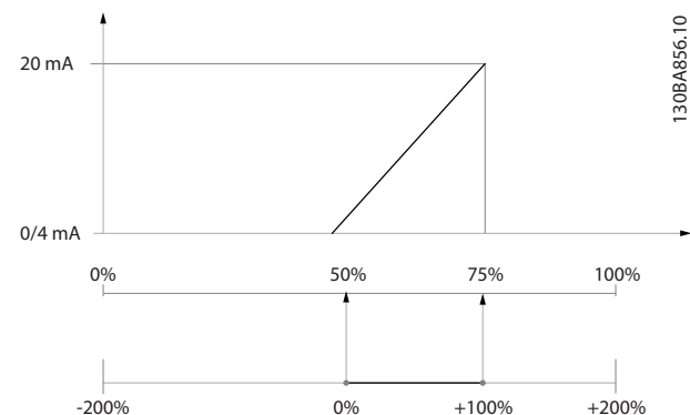
Рисунок 3.33 Пример 2
