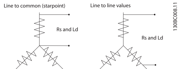
Рисунок 3.6 Характеристики обмотки статора
