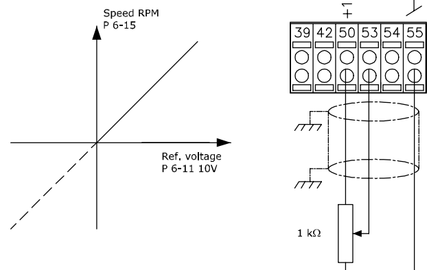
Рисунок 1.9 Задание от потенциометра
