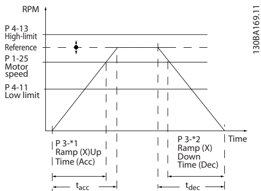
Рисунок 3.17 Изменение скорости 1
