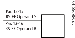
Рисунок 3.37 Триггеры сброса/установки
