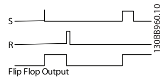
Рисунок 3.38 Выходы триггеров
