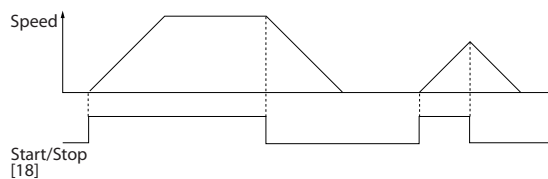
Рисунок 1.6 Пуск/останов
