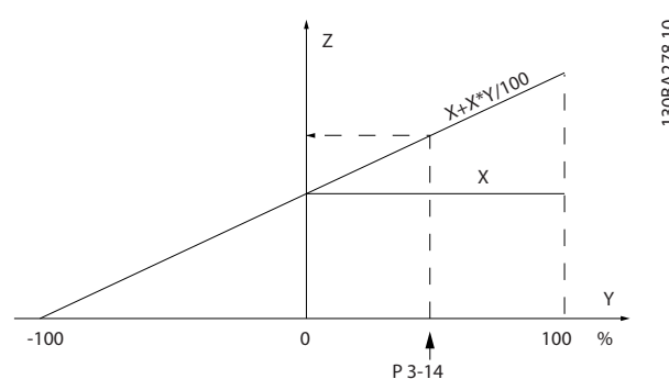
Рисунок 3.16 Фактическое задание
