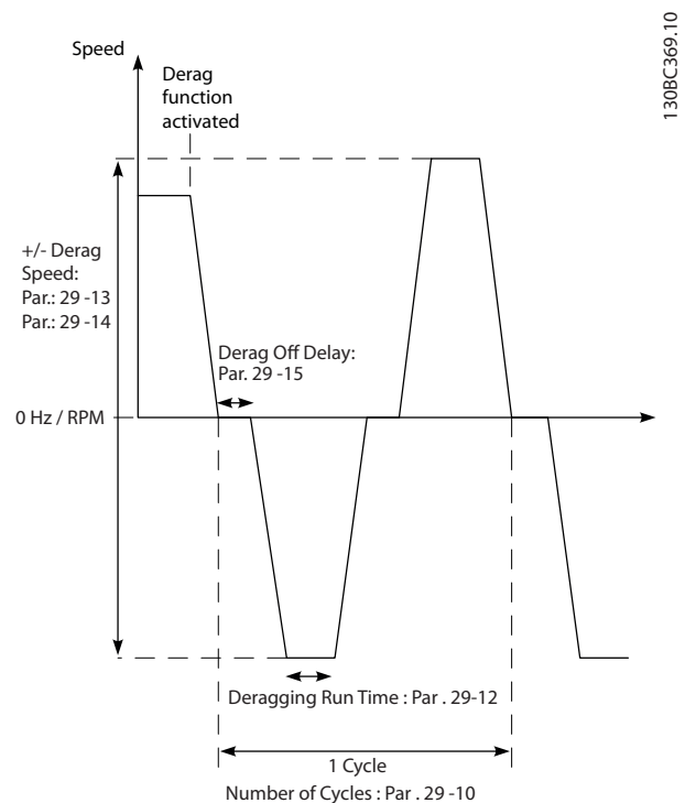
Рисунок 3.85 Функция очистки
