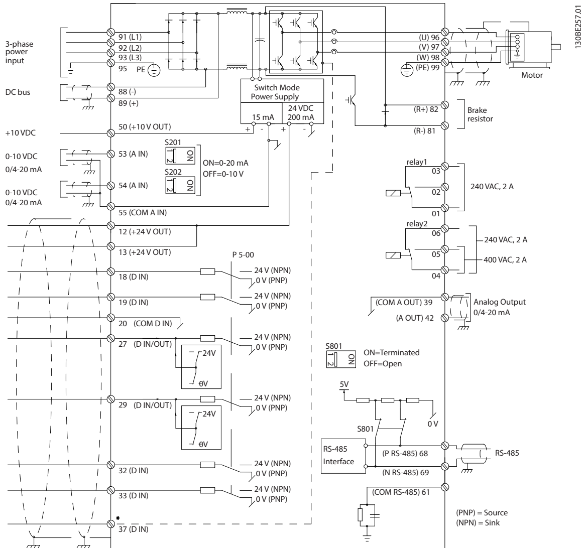
Рисунок 1.2 Схема основных подключений
