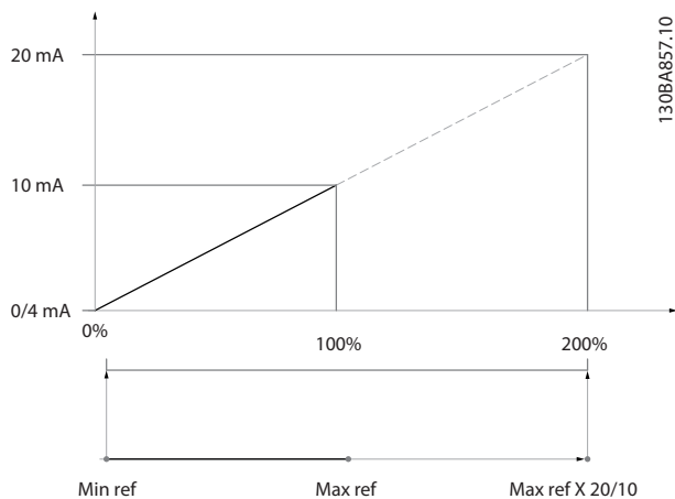
Рисунок 3.34 Пример 3
