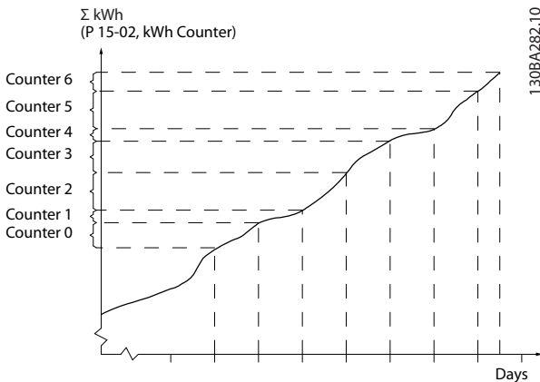
Рисунок 3.63 График энергопотребления
