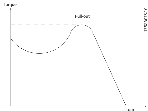
Рисунок 1.1 Момент опрокидывания
