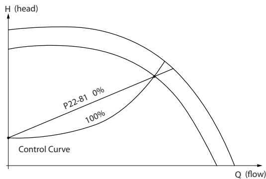
Рисунок 3.59 Квадратично-линейная аппроксимация характеристики
