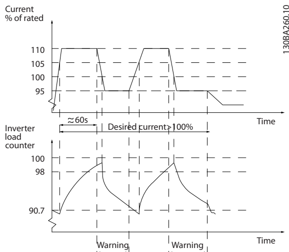
Рисунок 3.45 Выходной ток в условиях перегрузки
