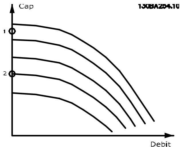
Рисунок 3.53 Диаграмма обнаружения отсутствия потока
