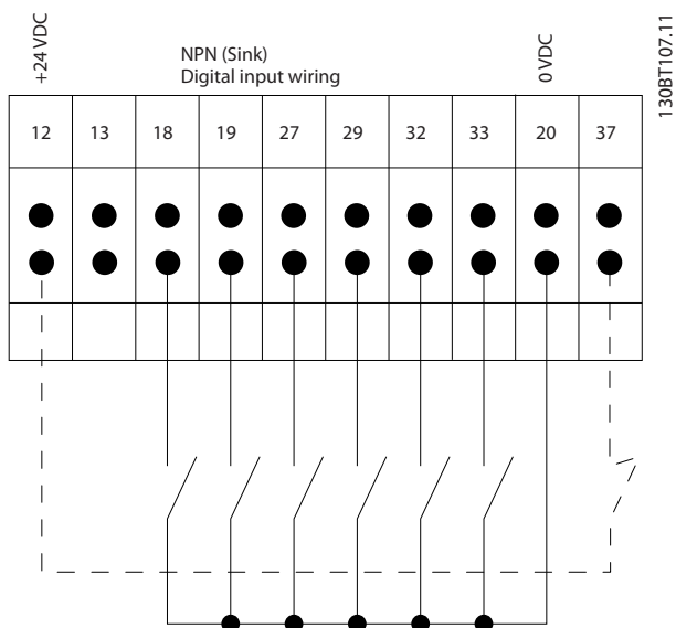
Рисунок 1.4 NPN (сток)
