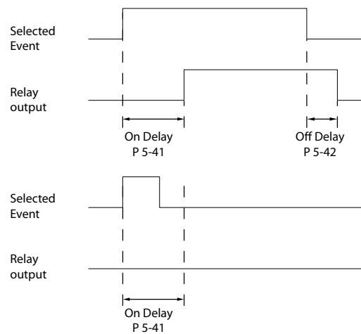
Рисунок 3.25 Задержка включения, реле
