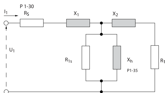
Рисунок 3.4 Эквивалентная схема асинхронного двигателя
