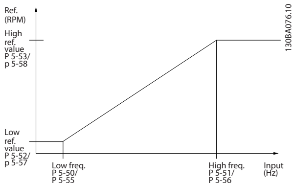
Рисунок 3.27 Импульсный вход
