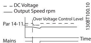
Рисунок 3.42 Кинетический резерв, короткое замыкание сети. Скачок происходит, пока в системе есть энергия.
