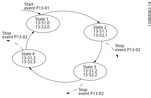
Рисунок 3.35 Действия событий интеллектуальной логики
