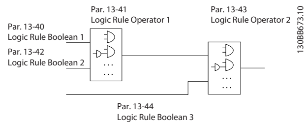
Рисунок 3.39 Логические соотношения
