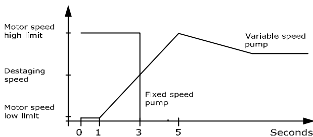
Рисунок 3.79 Порог выключения
