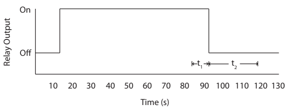
Рисунок 3.29 Пример выходной функции
