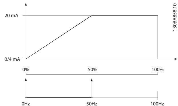
Рисунок 3.32 Пример 1
