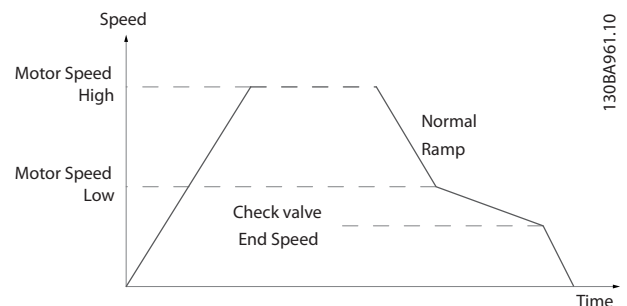
Рисунок 3.20 Изменение скорости контрольного клапана
