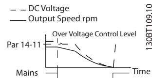
Рисунок 3.43 Кинетический резерв, более длительное замыкание сети. Двигатель останавливается выбегом, как только энергия в системе падает слишком низко.
