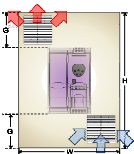
Размеры вентилируемого металлического шкафа (мм)
