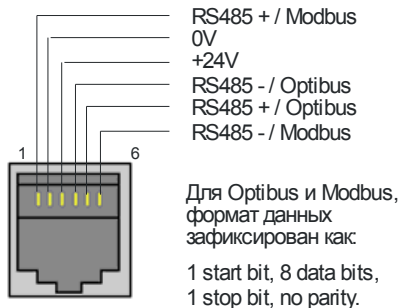
Rs485 интерфейс
