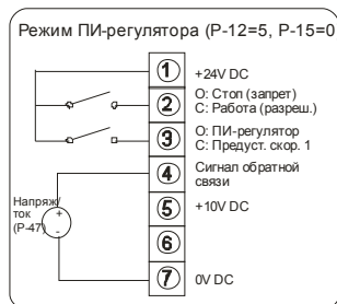
Режим ПИ-регулирования и предустановленная скорость 1
