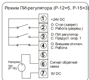
Режим ПИ-регулирования, предуст. скорость 1 и термистор двигателя
