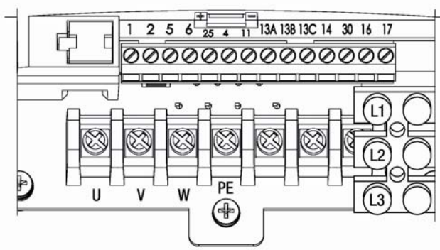
Трехфазная модель (3/PE) с фильтром 380 В переменного тока
