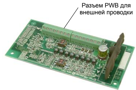
Плата обратной связи энкодера SJ-FB
