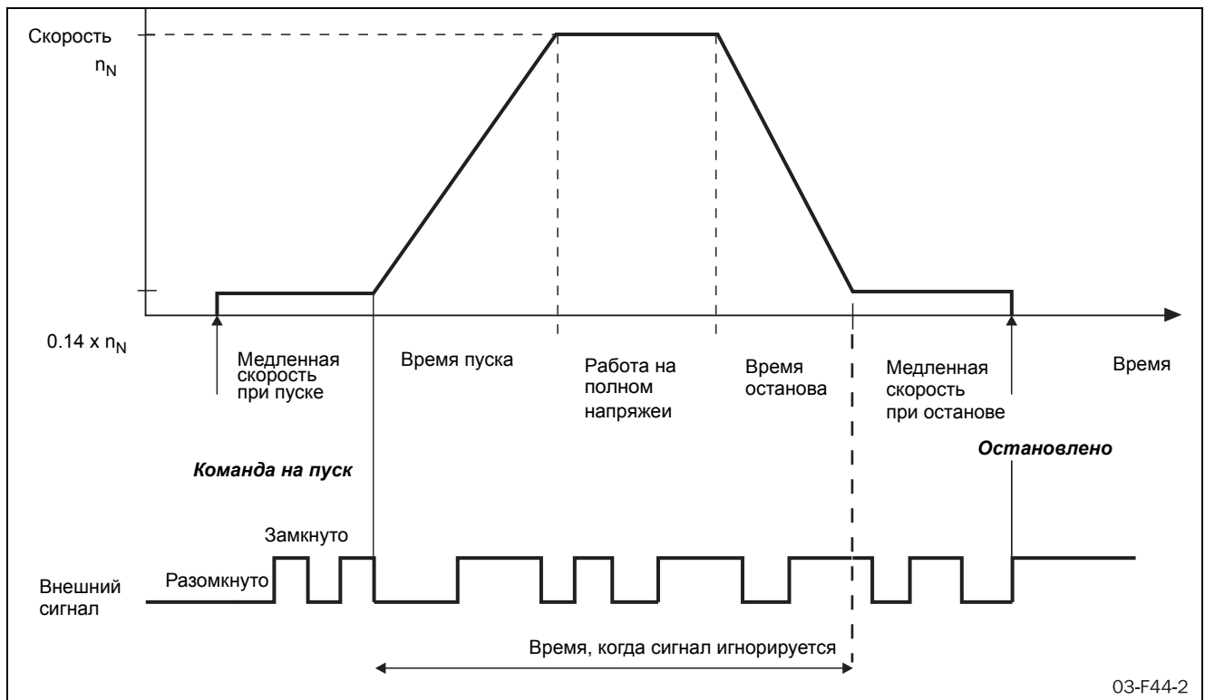
Рис. 46 Управление медленной скоростью при помощи внешнего сигнала
