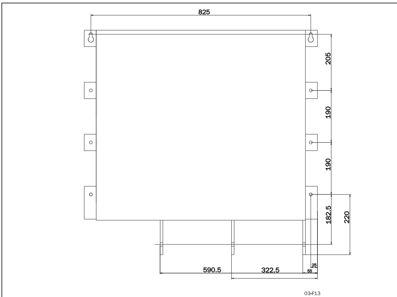
Рис. 18 Размеры отверстий для шин MSF-1000...MSF-1400
