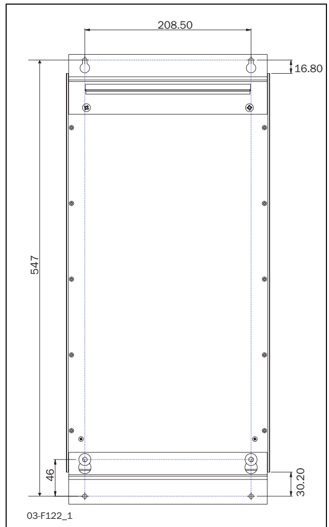
Рис. 16 Монтажные отверстия для MSF-170...MSF-250 с кронштейном верхнего крепления вместо DIN-направляющих.
