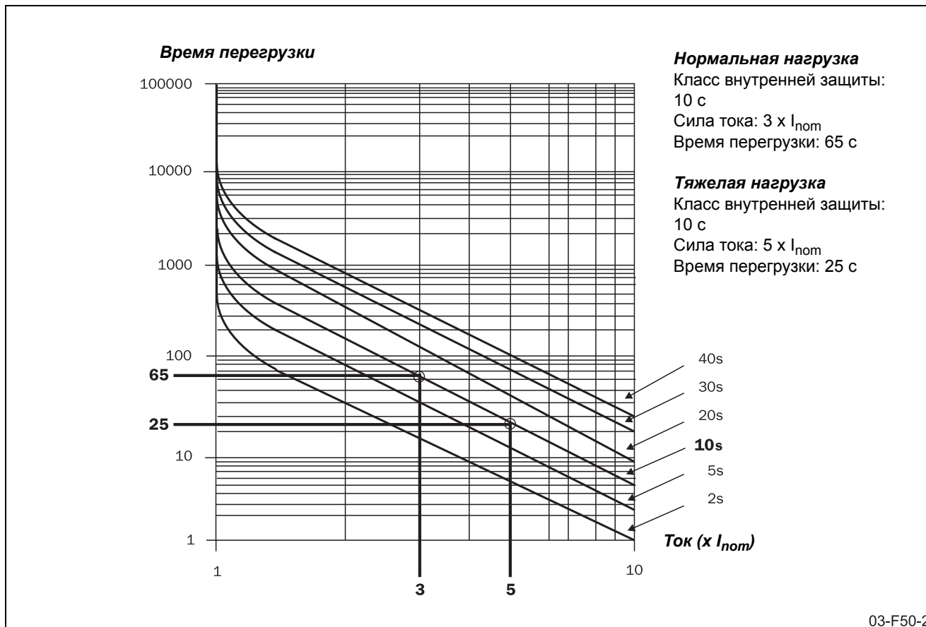
Рис. 34 Температурная кривая
