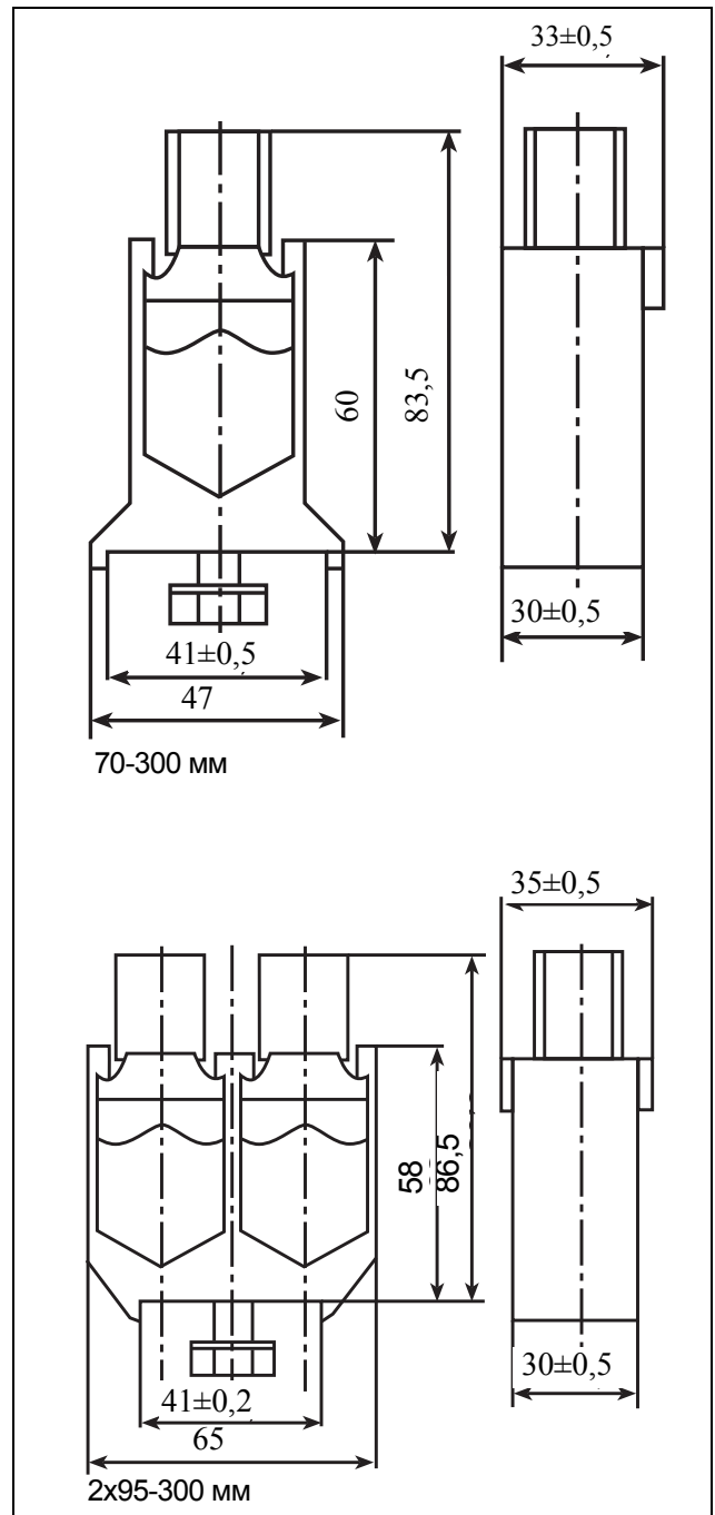
Рис. 74 Присоединительные клеммы
