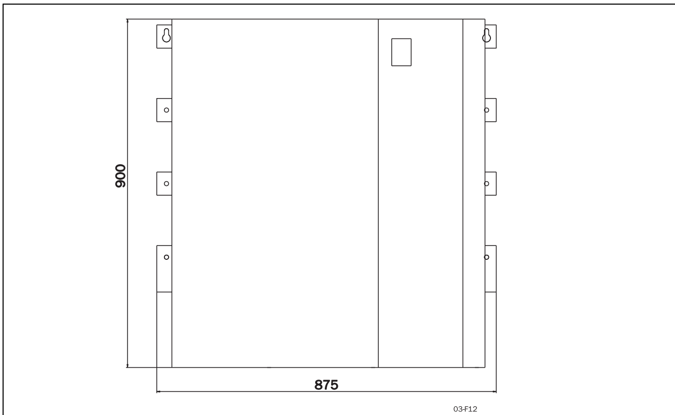
Рис. 17 MSF-1000...MSF-1400
