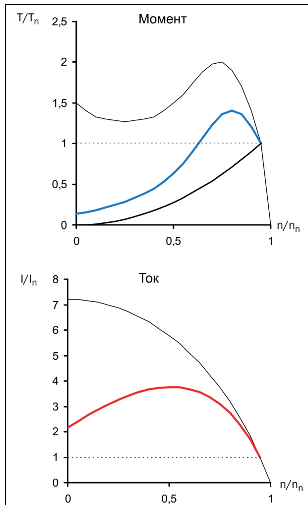
Рис. 8 Плавный пуск – плавное изменение напряжения
