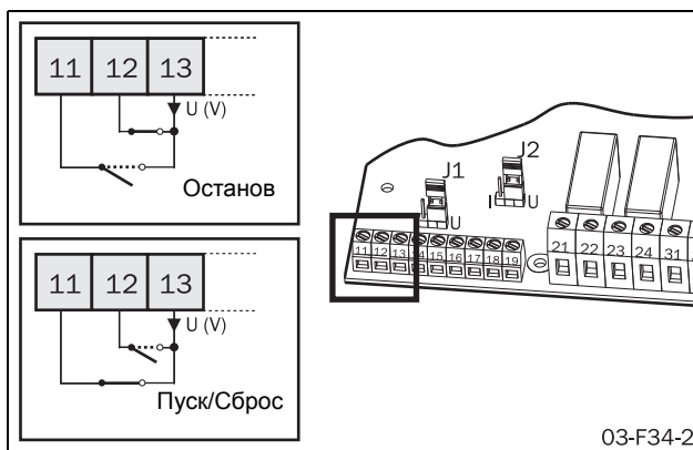
Рис. 64 3-проводной пуск/останов с автосбросом при пуске
