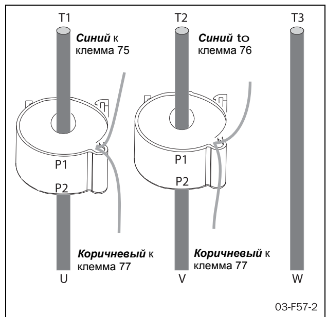
Рис. 51 Расположение трансформаторов тока при шунтировании на MSF-310 ... MSF-1400.
