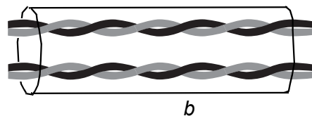
б Кабель, содержащий несколько витых пар в общем экране
