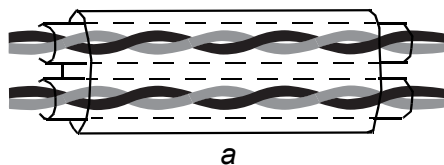
а Кабель, содержащий несколько витых пар в двойном экране
