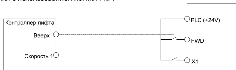
Рисунок 3. Нормальное соединение с использованием беспотенциальных контактов контроллера лифта.
