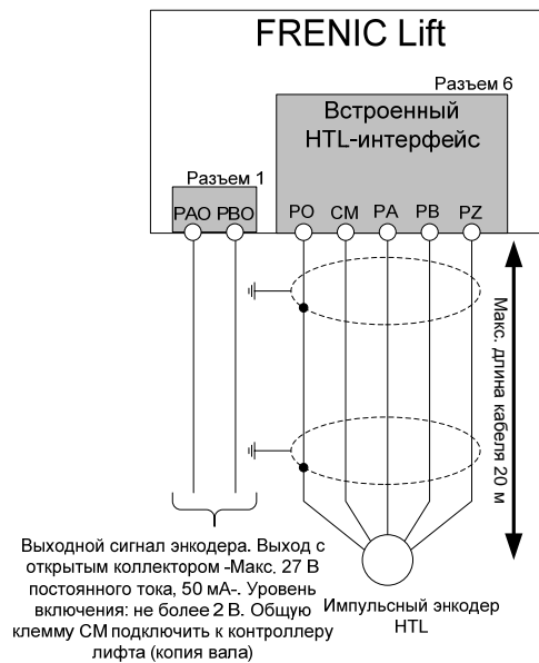
Рисунок 8. Соединение с помощью HTL-интерфейса энкодера.
