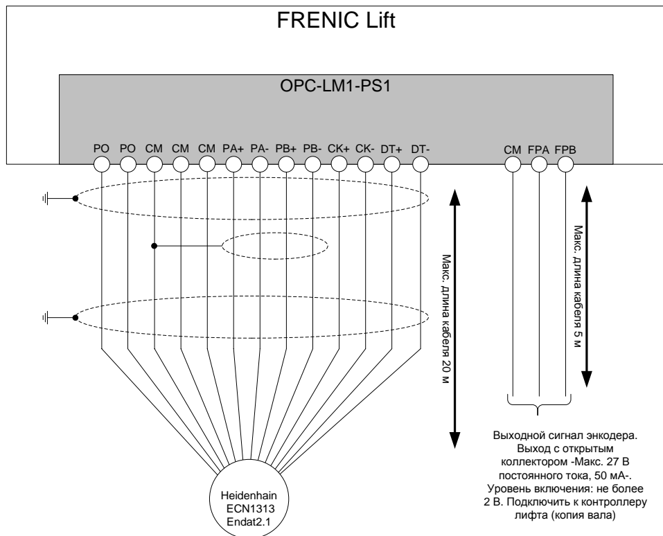
Рисунок 10. Соединение с дополнительной платой OPC-LM1-PS1.
