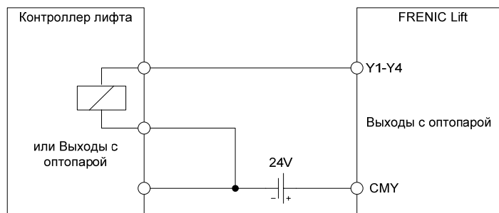
Рисунок 5. Соединение с использованием отрицательной логики PNP.
