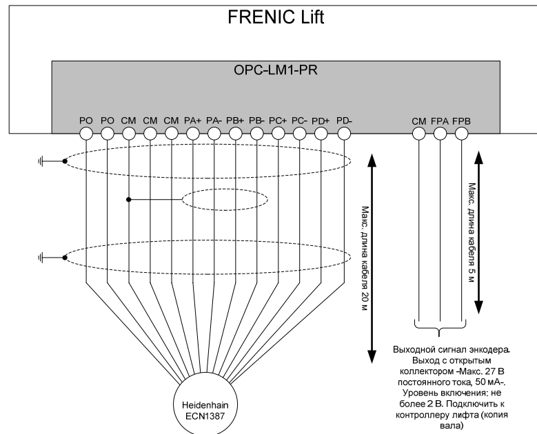
Рисунок 11. Соединение с дополнительной платой OPC-LM1-PR
