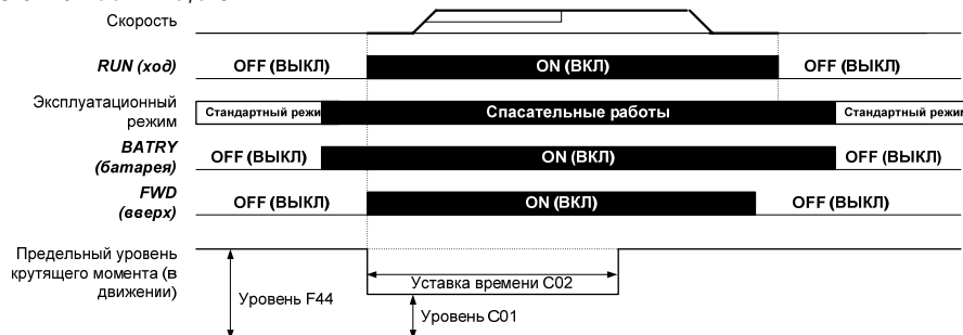
Рисунок 30. Работа на батареях с использованием функции ограничения крутящего момента.
