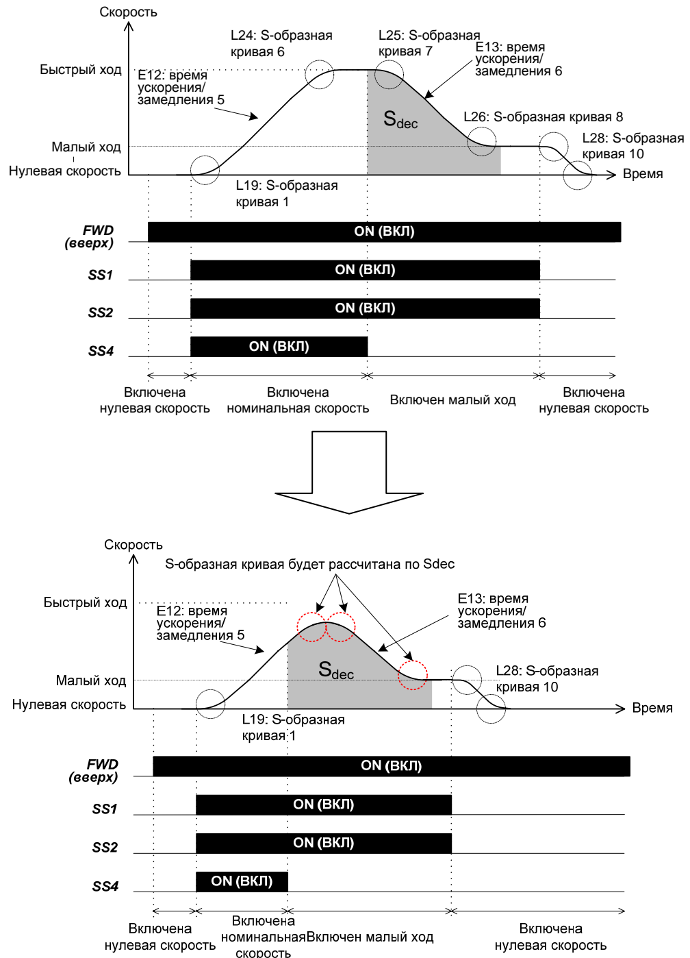
Рисунок 28. Короткие перемещения с постоянным регулированием пути.
