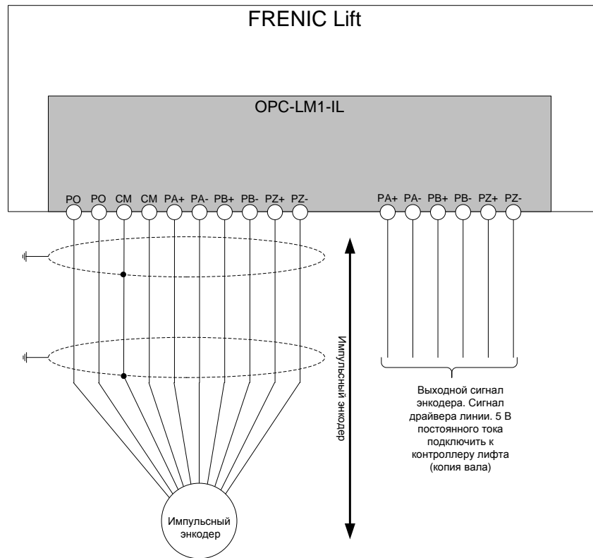
Рисунок 9. Соединение с дополнительной платой.
