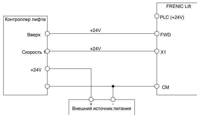
Рисунок 4. Соединение с использованием внешнего источника питания.
