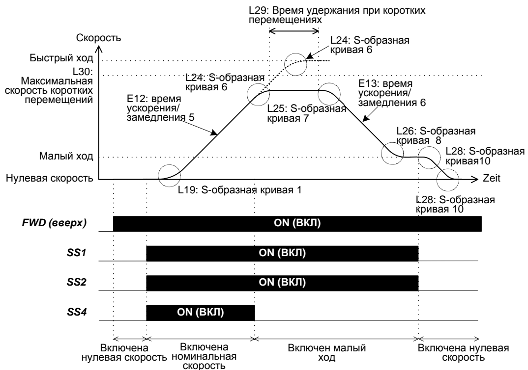
Рисунок 27. Классические короткие перемещения (регулирование частоты и времени).
