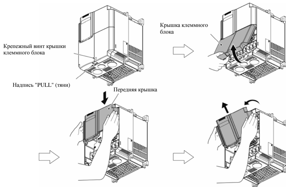
Рисунок 1. Снятие крышки клеммного блока и передней крышки.
