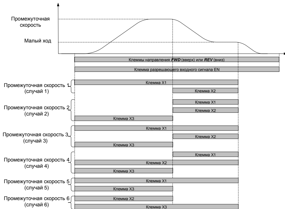
Рисунок 23. Временная диаграмма сигнала для перемещения с использованием промежуточных скоростей.
