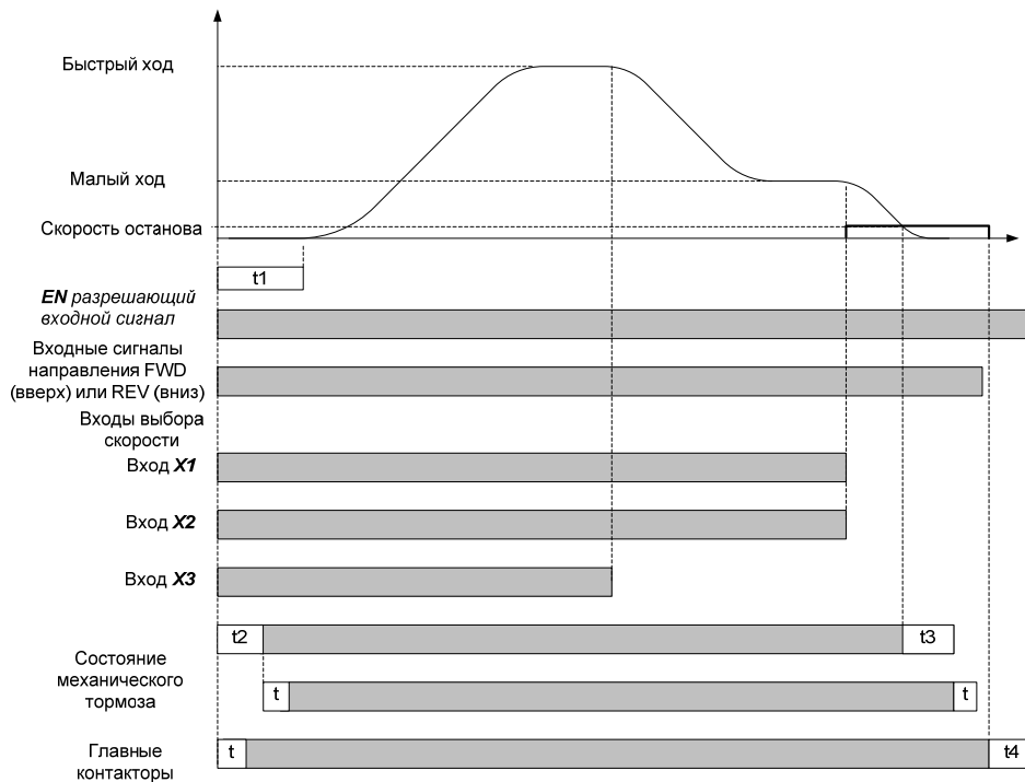
Рисунок 22. Временная диаграмма сигнала для нормального перемещения.
