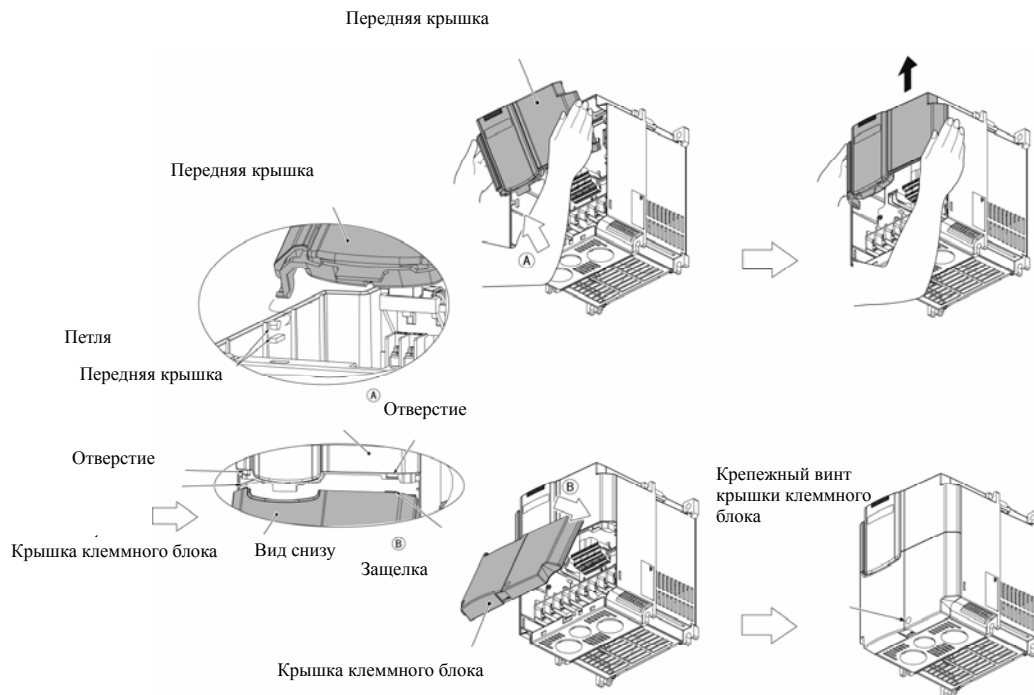
Рисунок 1. Снятие крышки клеммного блока и передней крышки.
