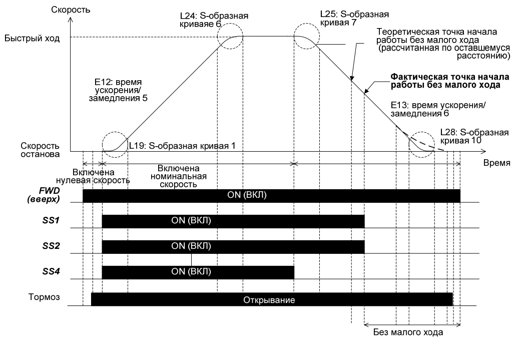
Рисунок 29. Работа без малого хода.
