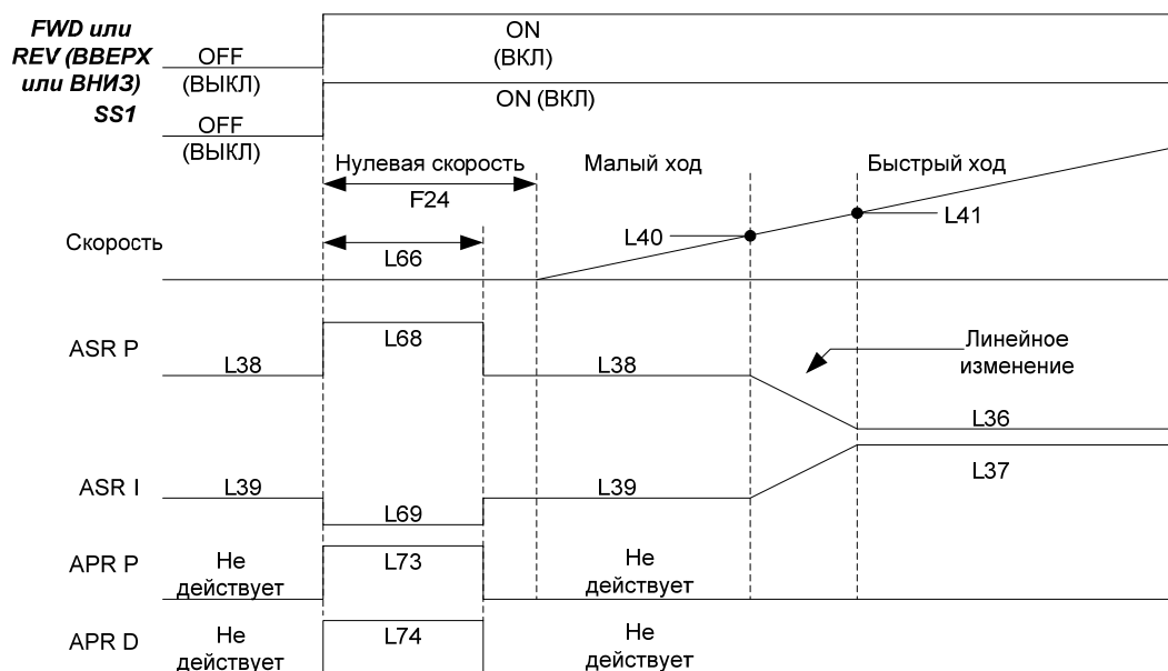
Рисунок 26. Временная диаграмма с выравниванием несимметричной нагрузки (L65 = 1).
