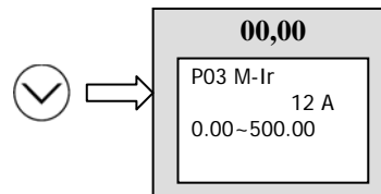
Рисунок 21. Изменение значения P03 (номинальный ток двигателя). В данном случае на 12.
