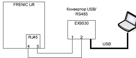
Рисунок 7. Соединение FRENIC Lift с ПК
