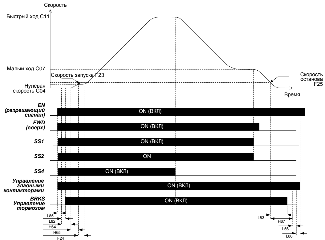
Рисунок 31. Временная диаграмма сигнала при использовании функции плавного пуска.
