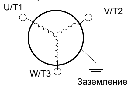
3 фазный электродвигатель переменного тока.
