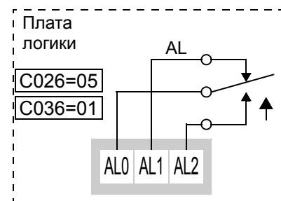
Реле при включенном инверторе, сигнала Аварии нет
