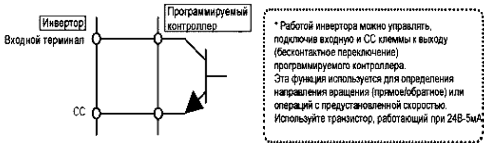
* Соединение инвертора с программируемым контроллером
