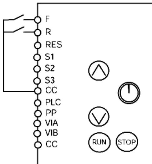
CMoD = 0 (Входные терминалы)
