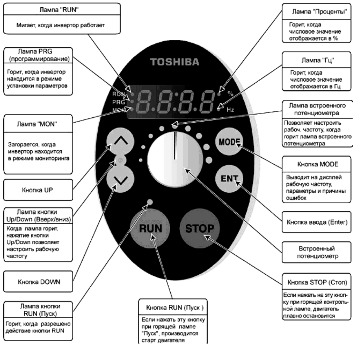
(Передняя панель 1)
