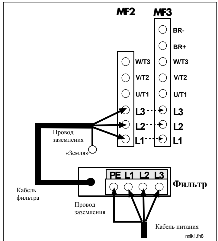
Рис. 6-11. Подключение кабелей при установке фильтра радиочастотных помех в Vacon NXL
