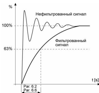
Рисунок 9.7: Фильтрация сигналов A11 и A12
