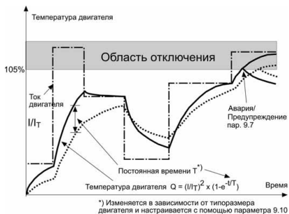
Рисунок 9.9: Расчет температуры двигателя
